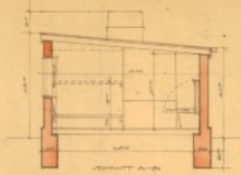
MAßSTAB 1:40
