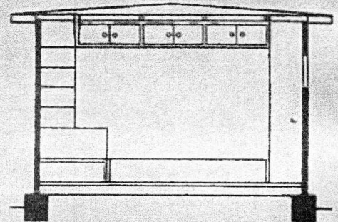
SCHNITT E-F
