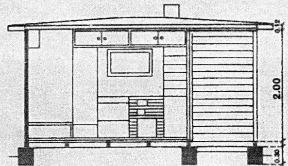
SCHNITT A-B
